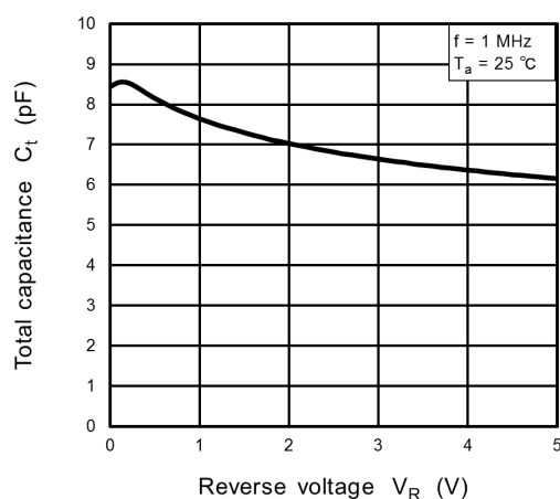
Fig. 8.3 C_t - V_R
