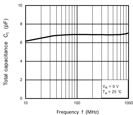
Fig. 8.4 C_t - f
